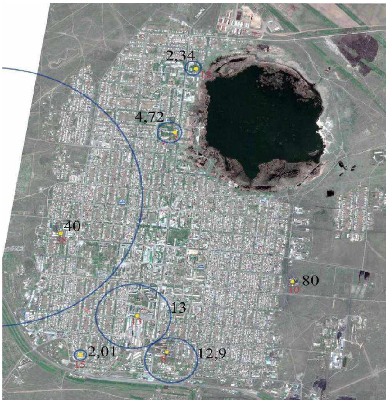
Рисунок 1.1 – Расположение источников тепловой энергии и их существующие зоны действия на территории муниципального образования муниципальный округ город Славгород Алтайского края
