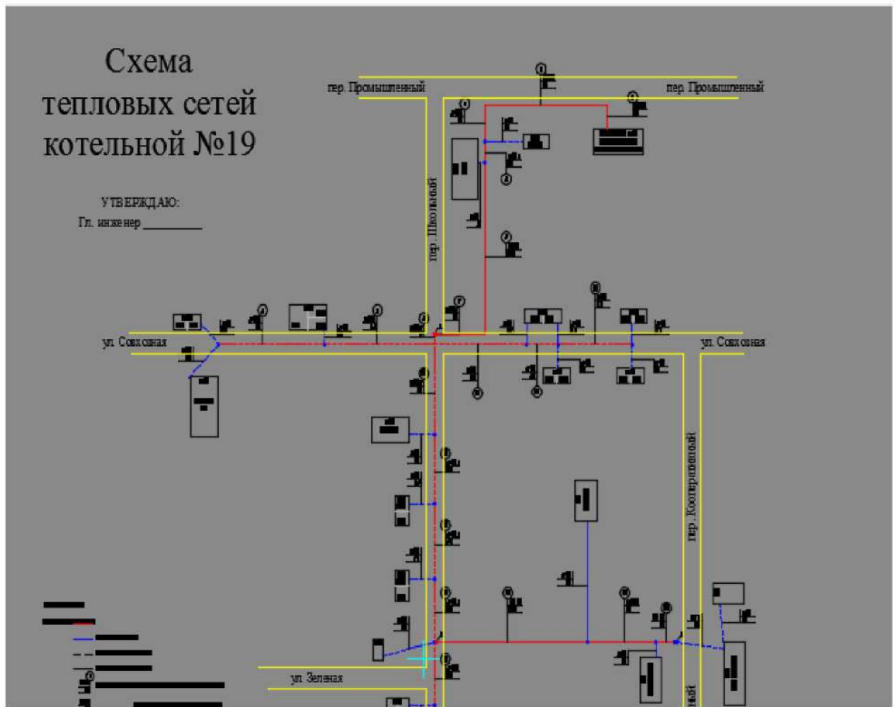
Схемы тепловых сетей в зоне действия источника тепловой энергии Котельная 19 г. Славгород (с. Нововознесенка ул. Промышленная)
